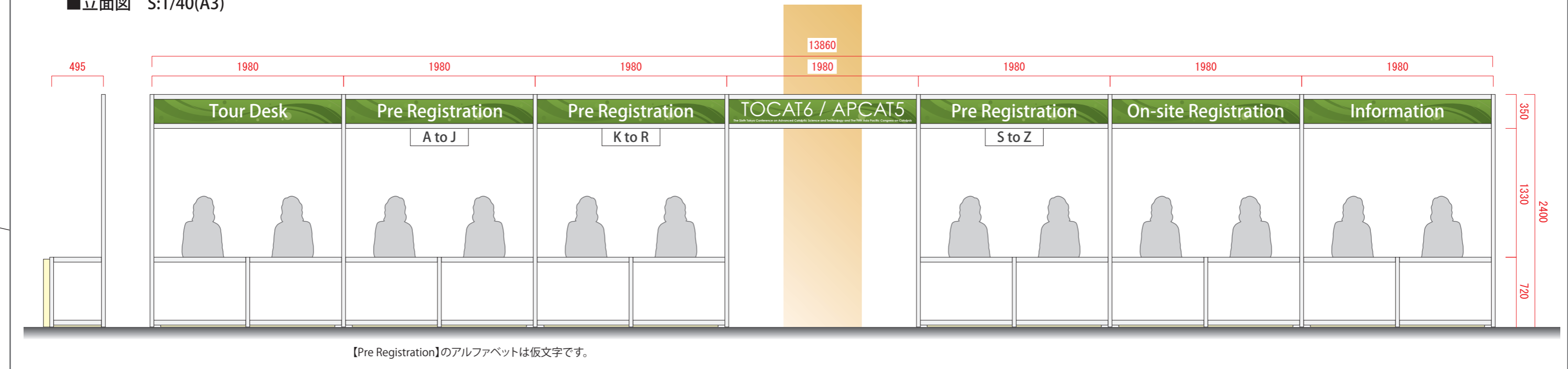
■立面図 S:1/40(A3)
